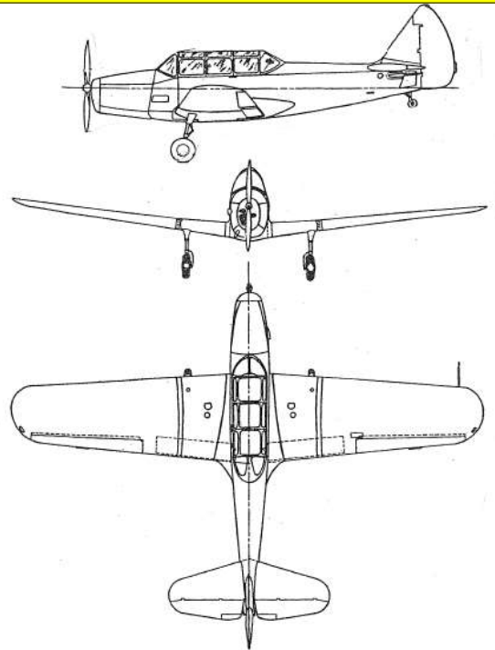
PT-26 "CORNELL" M-62A-3 N9474H
